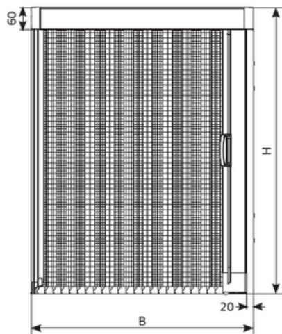
montaż: wnęka okienna
