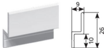
profil prowadnicy typ „Z”
