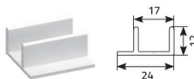
profil prowadnicy typ „U”
