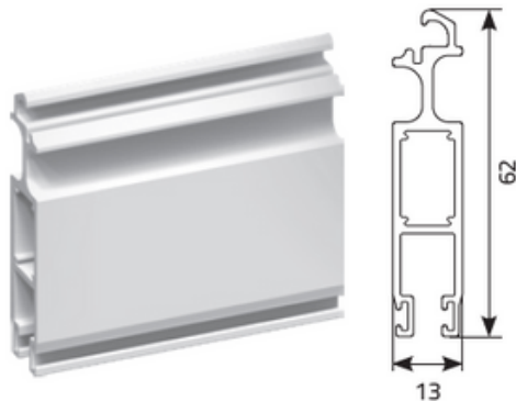
profil ramki „MPR”
