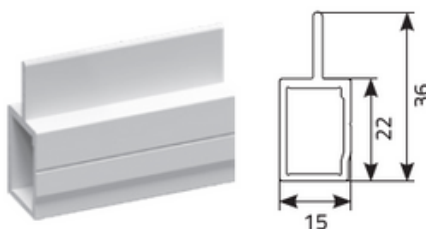
profil prowadnicy typ „F1”
