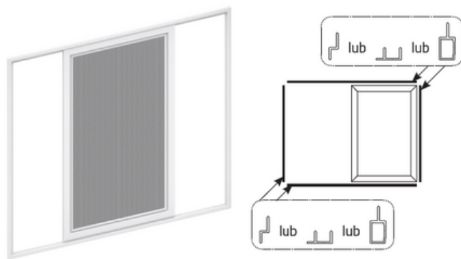
Moskitiera jednoskrzydłowa z futryną
