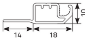
Przekrój profilu MR-1
