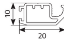
Przekrój profilu MR-2
