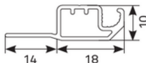
Przekrój profilu MR-1
