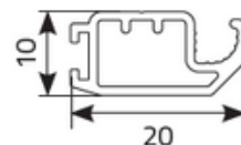
Przekrój profilu MR-2
